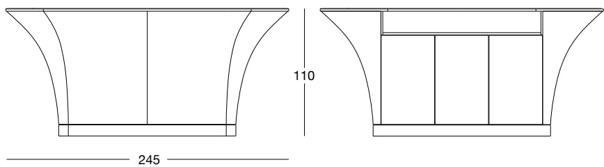
Piano acciaio senza vaschetta con scarico Wash-basin without drain-pipe Раковина без слива
